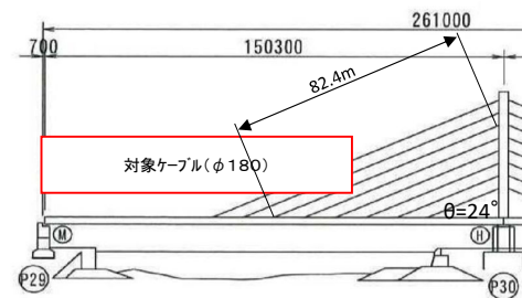
＜斜張橋＞
