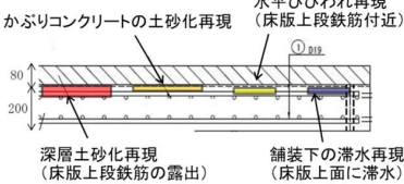
断面構成
